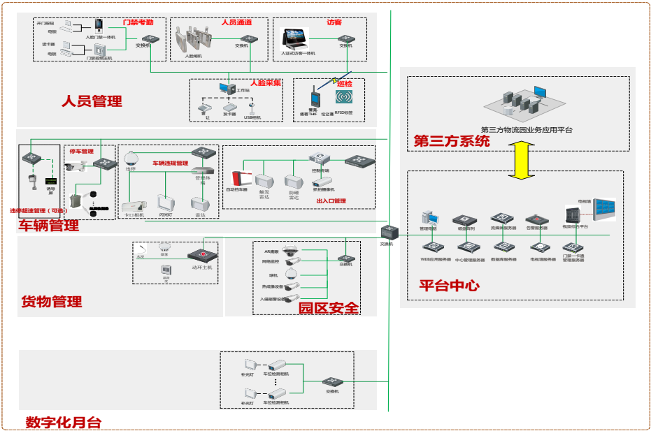
系统拓扑
