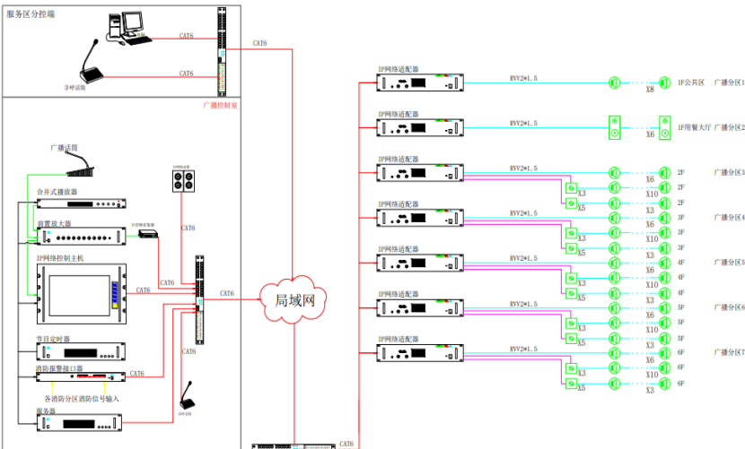
综合楼广播系统图
